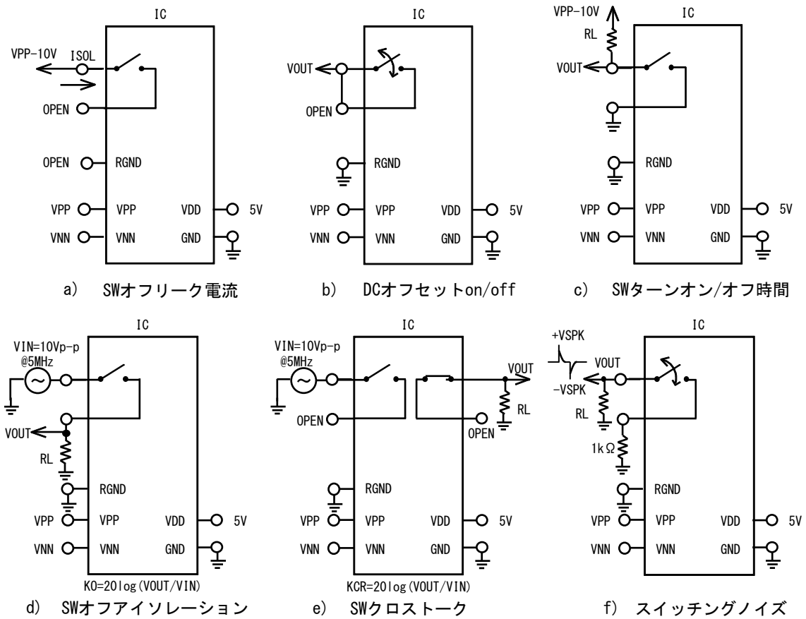
図 4.1 測定回路
