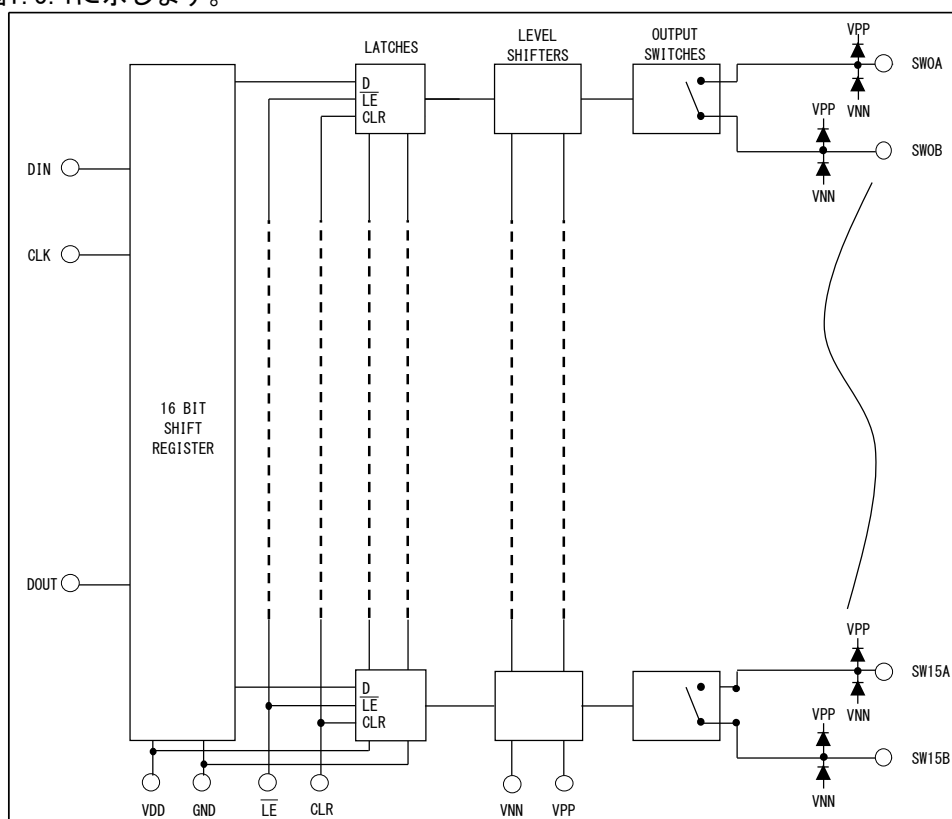
図1.3.1 回路ブロック
