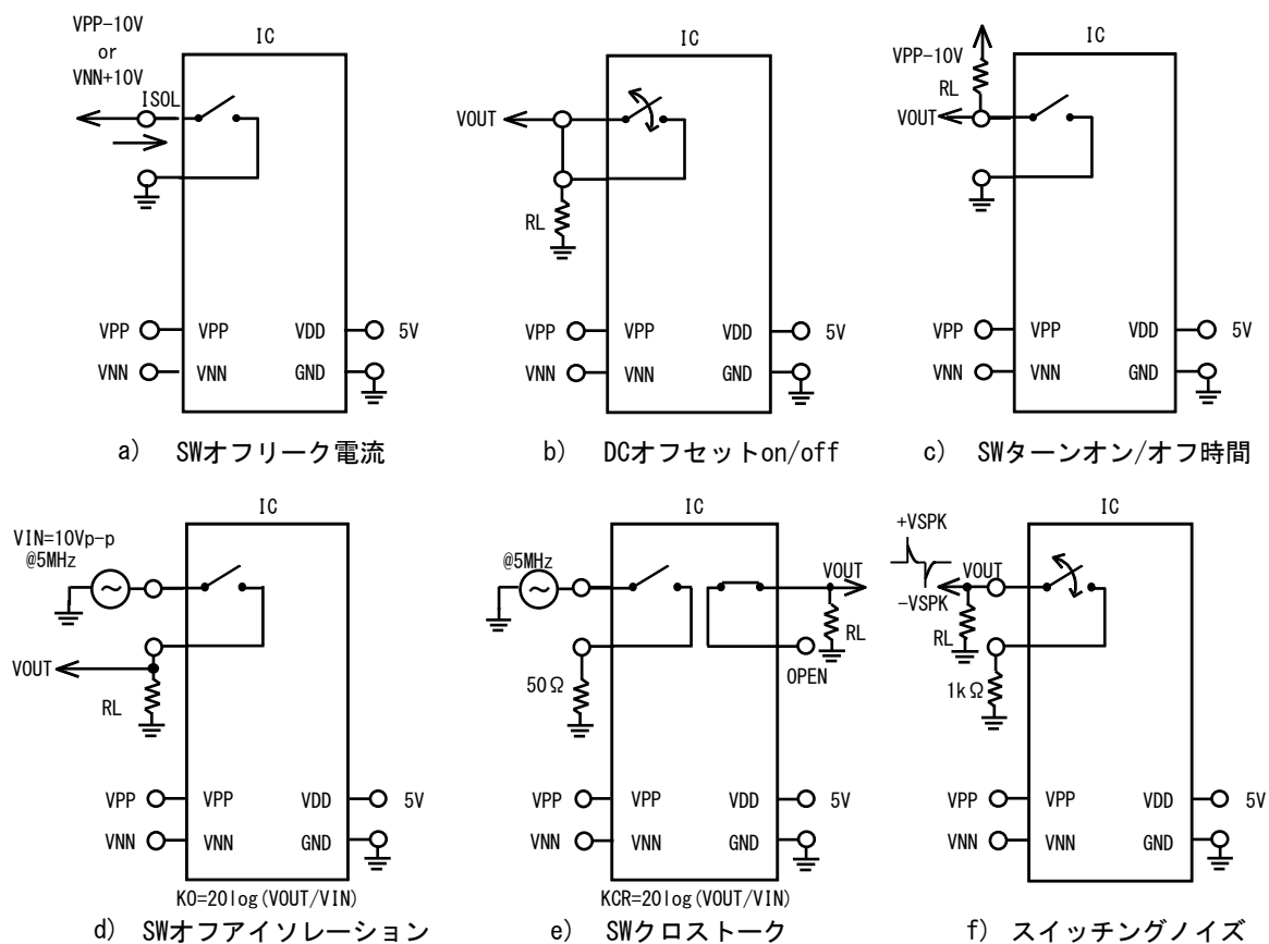
図 4.1 測定回路
