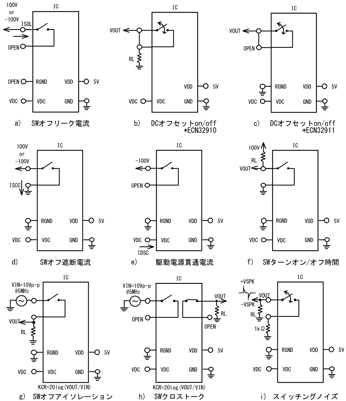
図 4 測定回路
