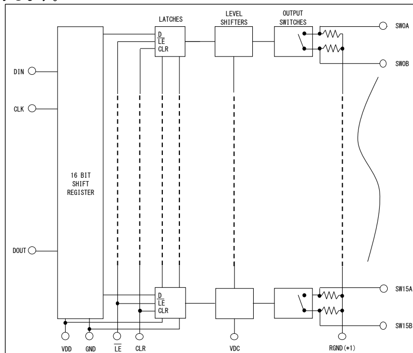
図1.3.1 回路ブロック
