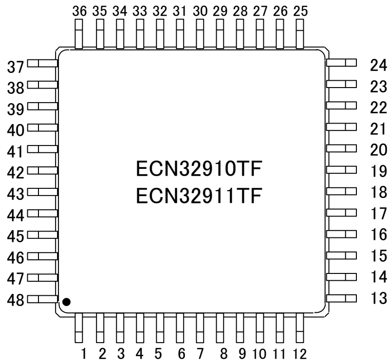
図8.1 端子配置（上面）
