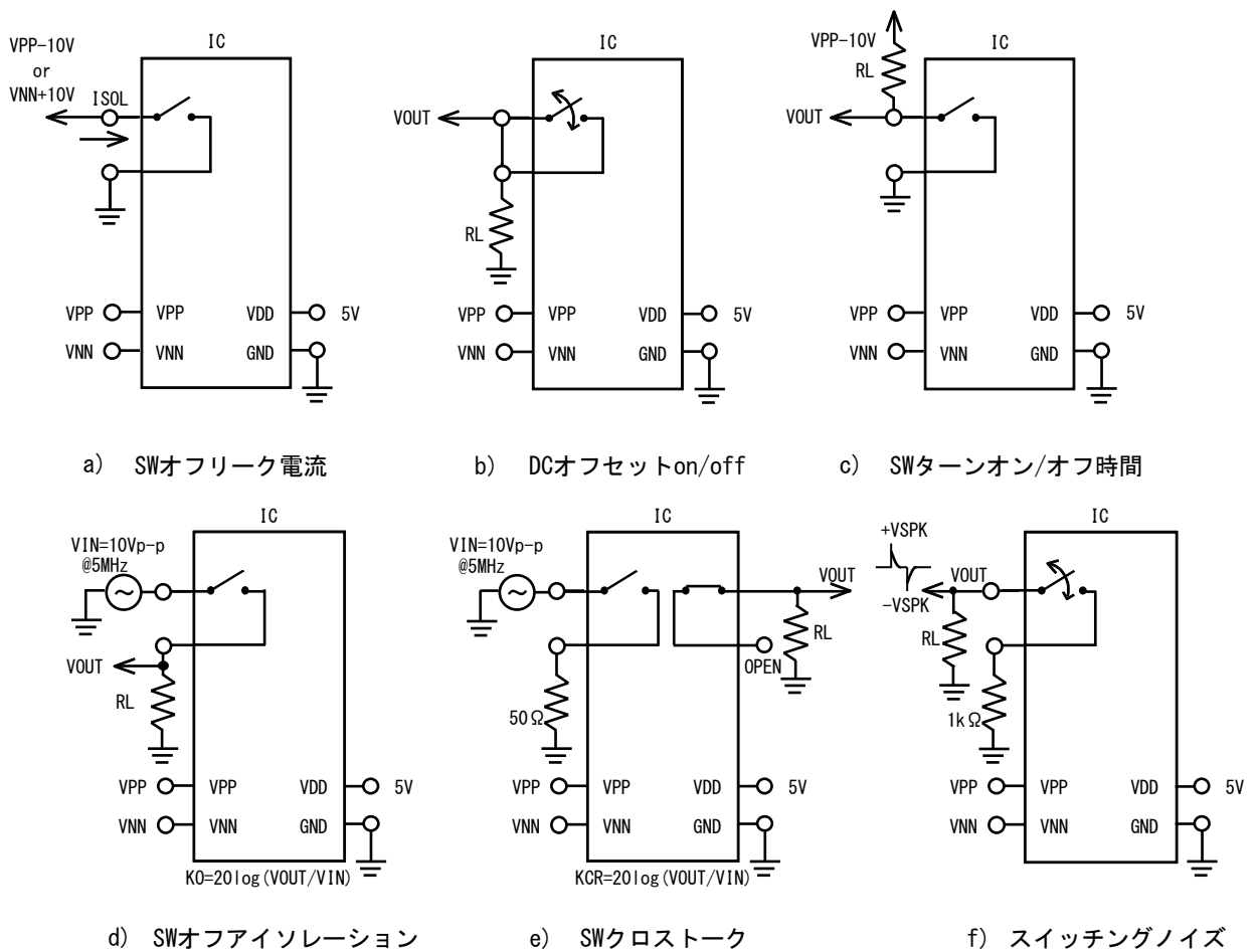
図 4.1 測定回路
