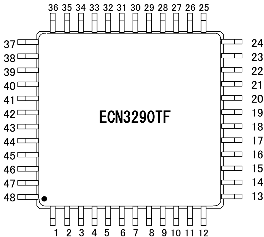
図8.1 端子配置（上面）
