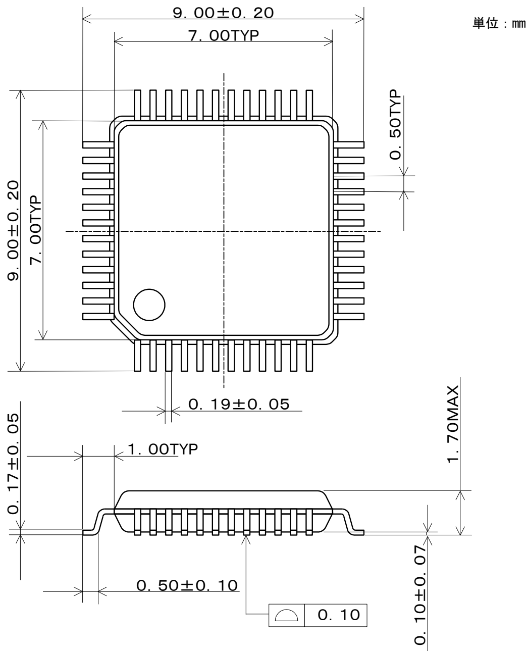
図A パッケージ外形寸法
