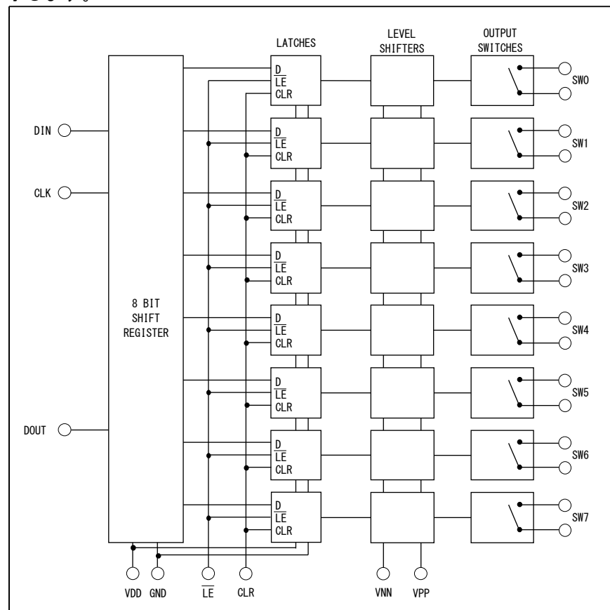
図1.3.1 回路ブロック
