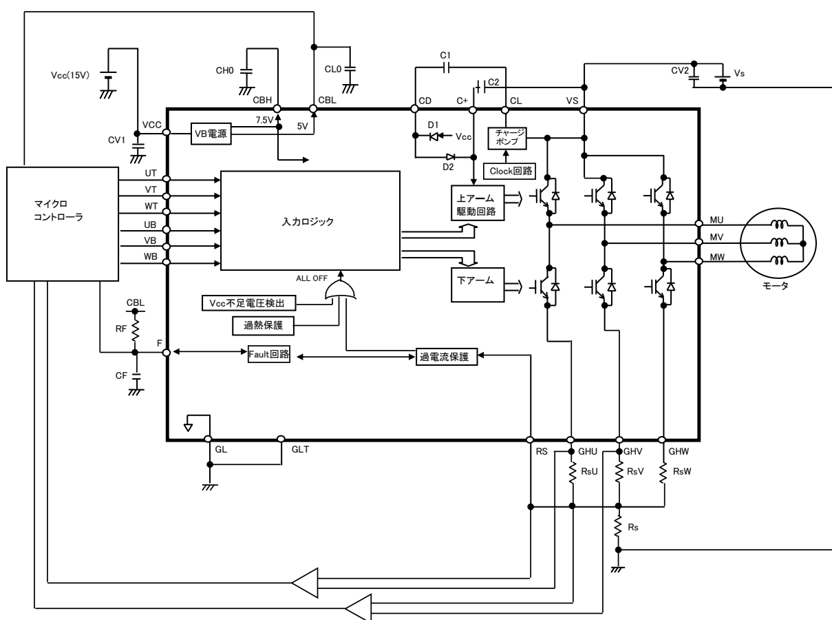
図3.1.1 回路ブロック (太枠内：ECN30632)
