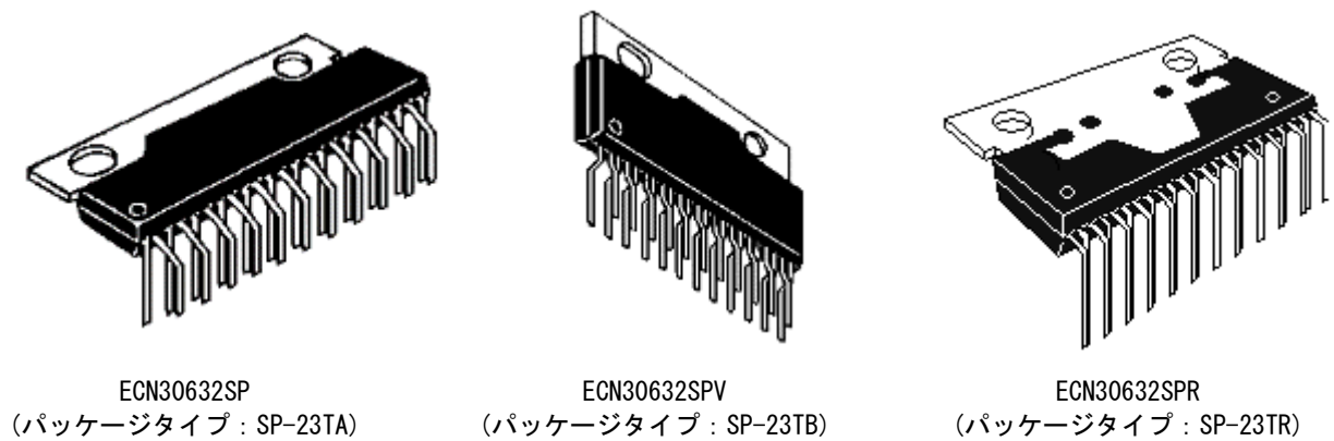
図1.4.1 ECN30632外形
