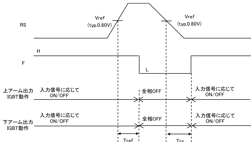
図 3.5.1.5 過電流保護動作時のタイミングチャート
