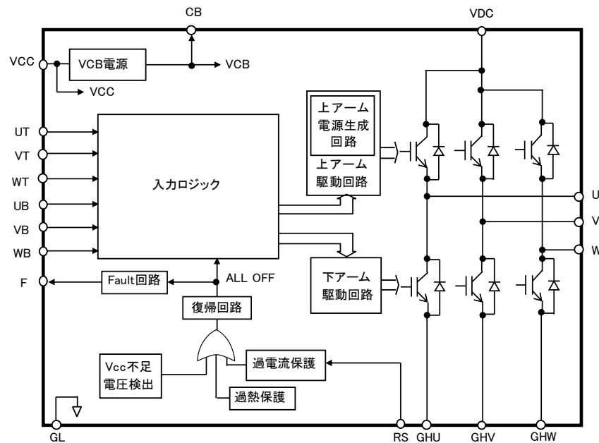
図 1.3.1 ICのブロック図
