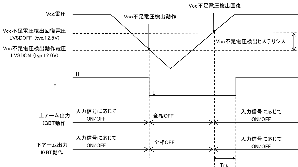
図 3.5.1.1 Vcc 不足電圧検出動作時のタイミングチャート
