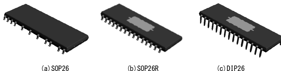
図 1.1.2 IC 外形図
