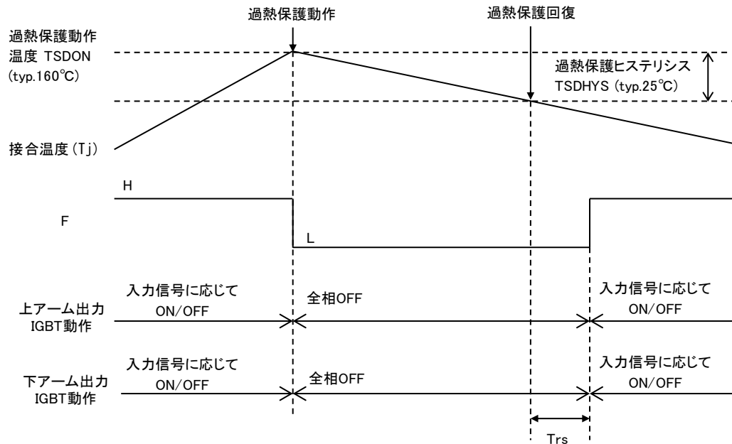
図 3. 5. 1. 6 過熱保護動作時のタイミングチャート
