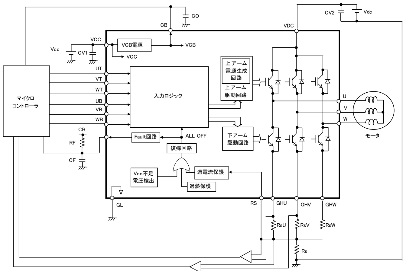
図 4.1.1 ICのブロック図と外付け部品
