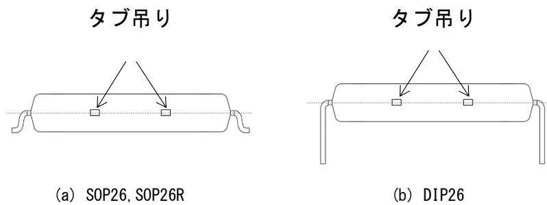
図 3.6.1.1 IC 側面図
