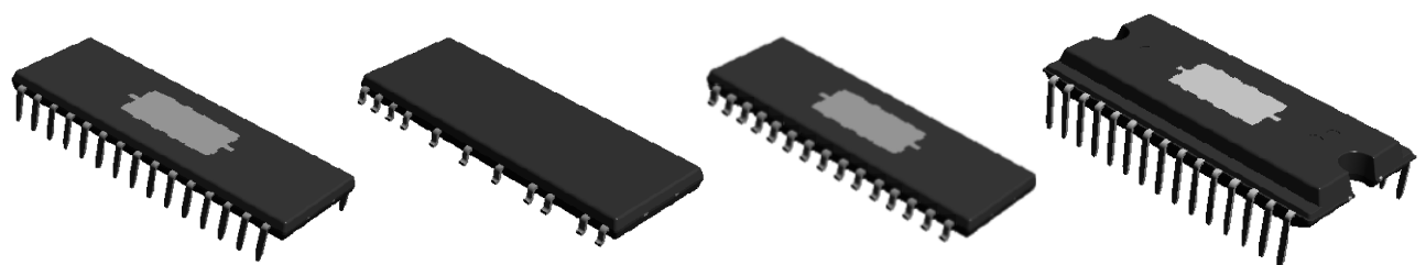
ECN30624P (パッケージタイプ : DIP26) ECN30624F (パッケージタイプ : SOP26) ECN30624R (パッケージタイプ : SOP26R) ECN30624PN (パッケージタイプ : DIP26N)
