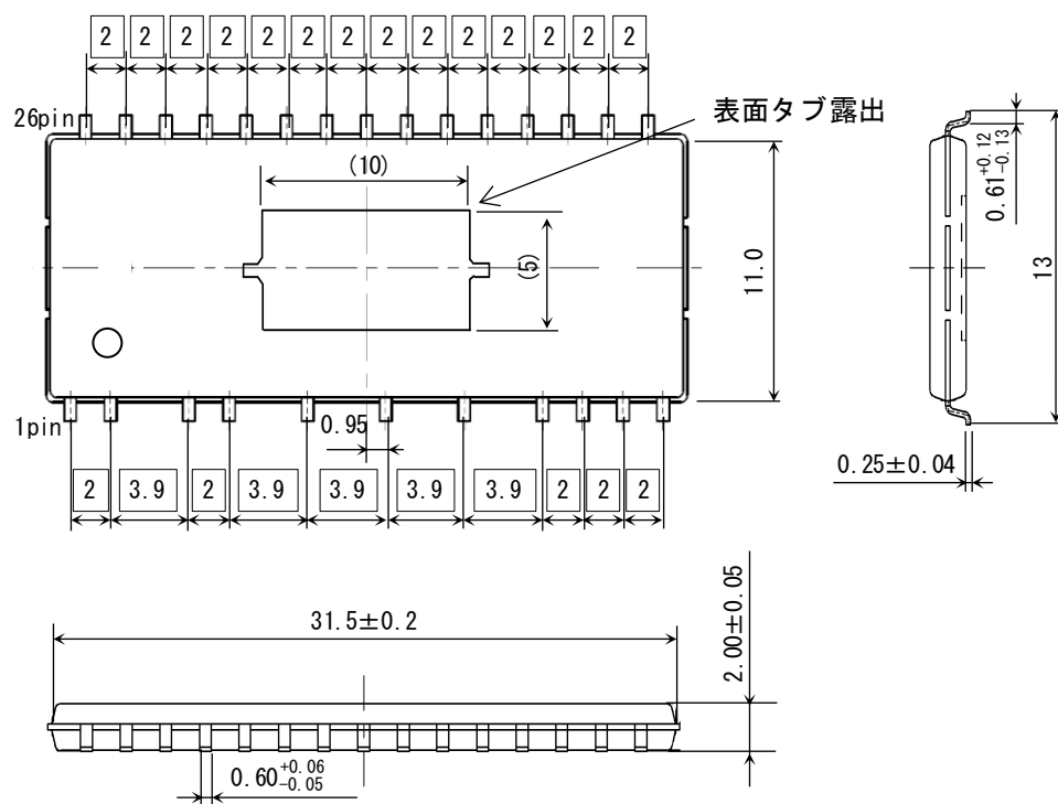
図C SOP26Rパッケージ外形寸法
