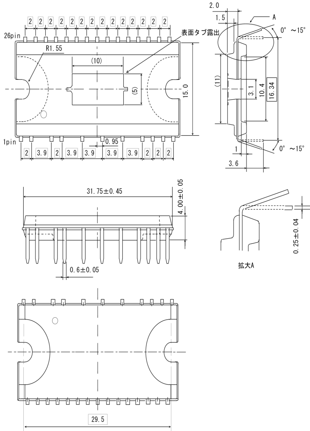
図D DIP26Nパッケージ外形寸法
