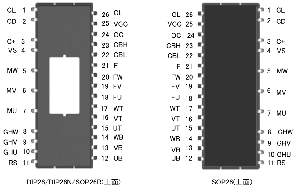
図5.1 端子配置
