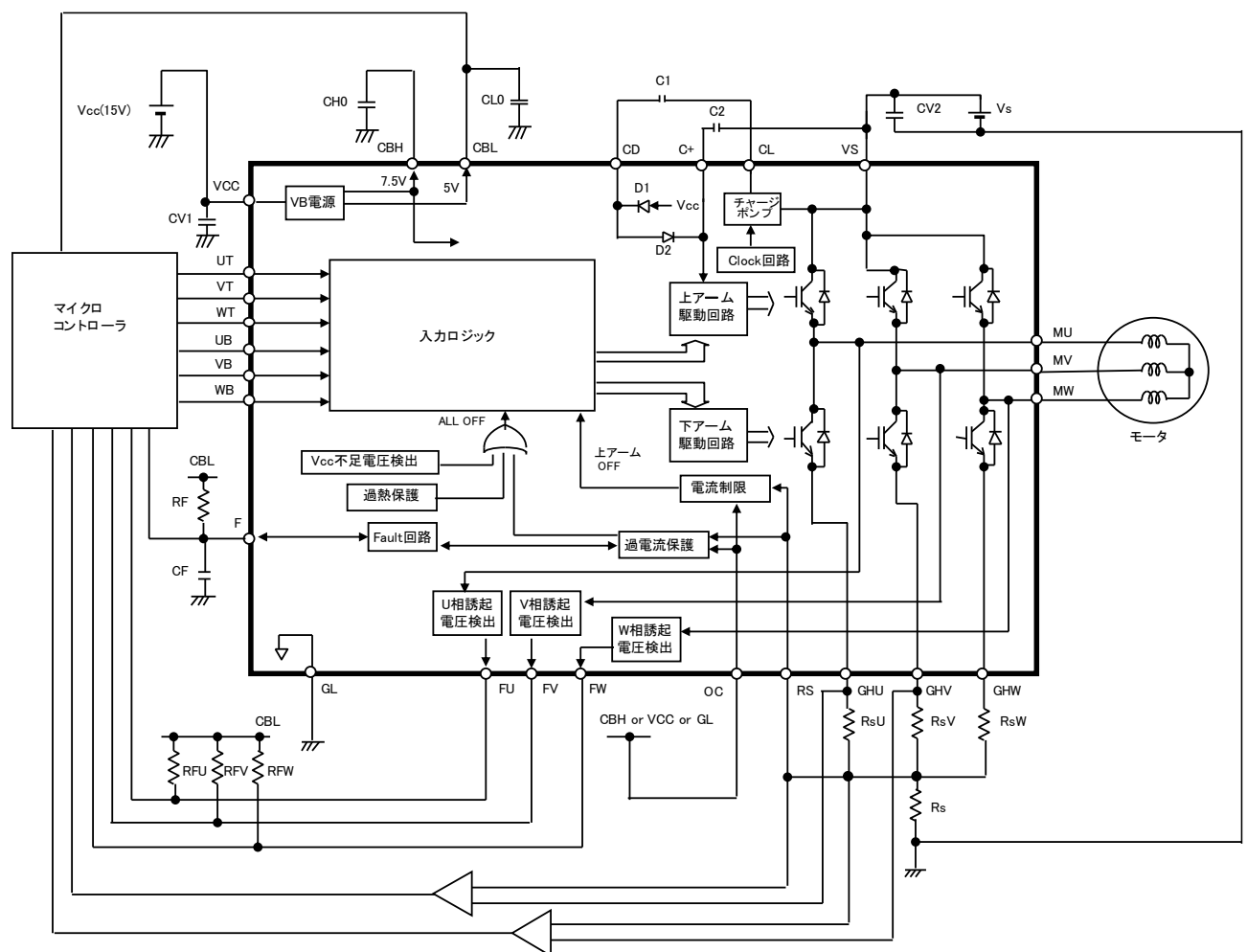
図3.1.1 回路ブロック (太枠内: EGN30622)
