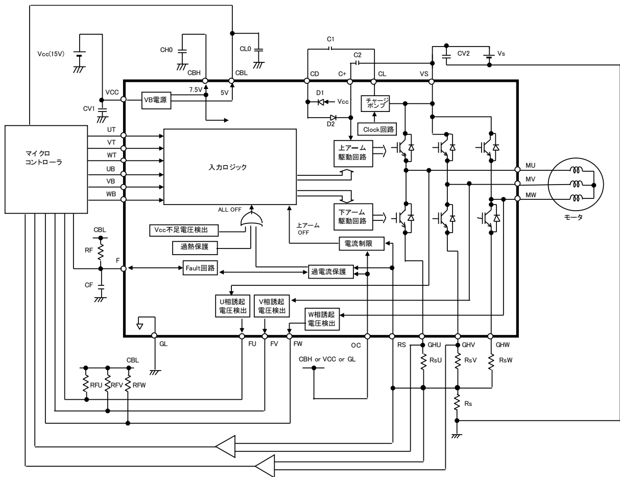
図3.1.1 回路ブロック (太枠内: EGN30620)
