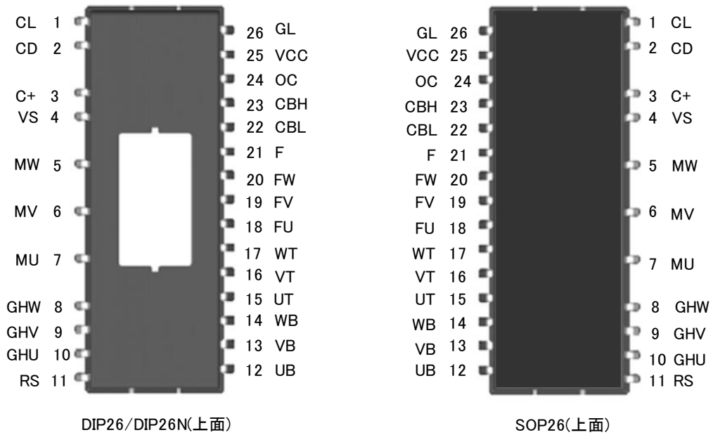
図5.1 端子配置
