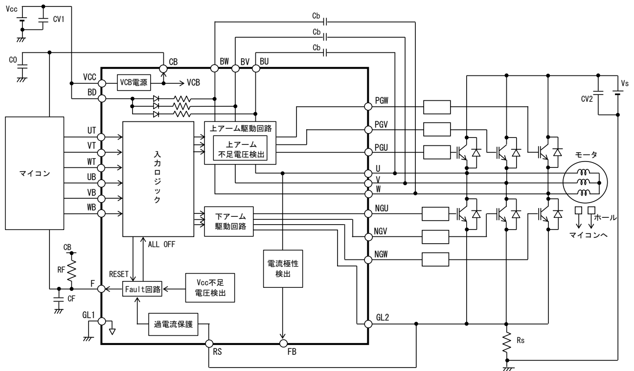
図3.1.1 ICのブロック図と外付け部品
