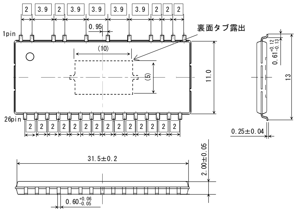
図B SOP26パッケージ外形寸法
