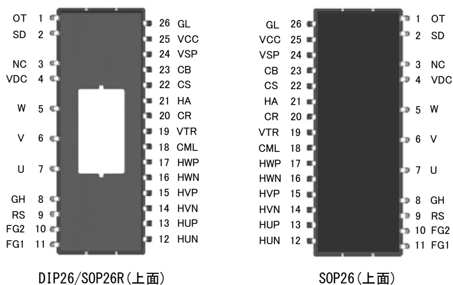
図5.1 端子配置
