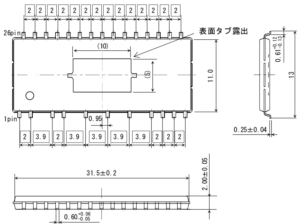
図C S0P26Rパッケージ外形寸法
