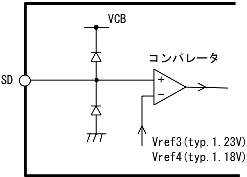
図2. 2. 6 SD端子の等価回路
