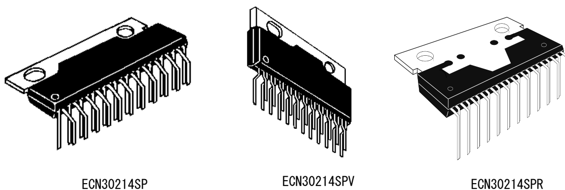
図1.4.1 ECN30214の外形
