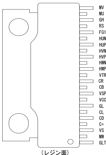
図5.1 端子配置
