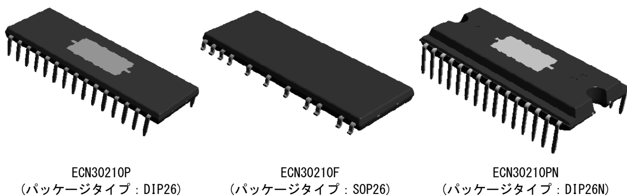
図1.4.1 EGN30210の外形
