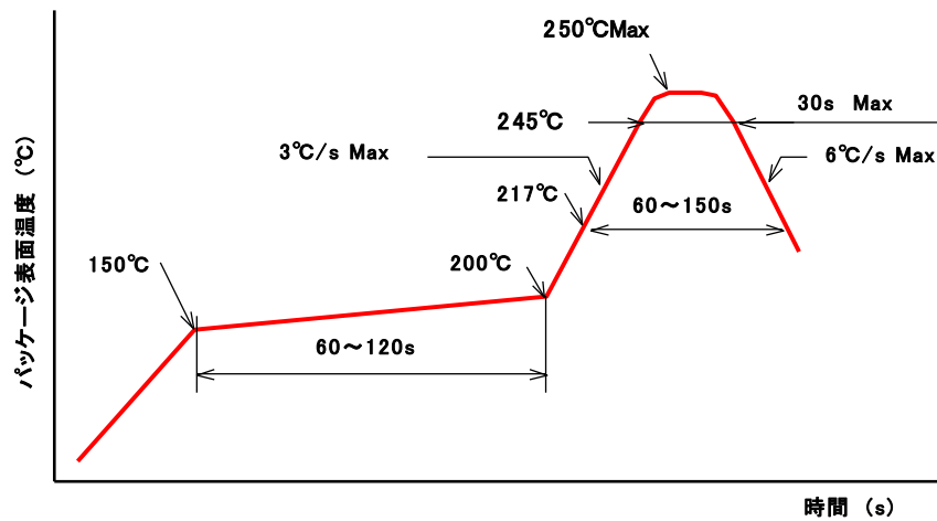
図8.7.1 赤外線リフローおよびエアールフロー推奨条件
