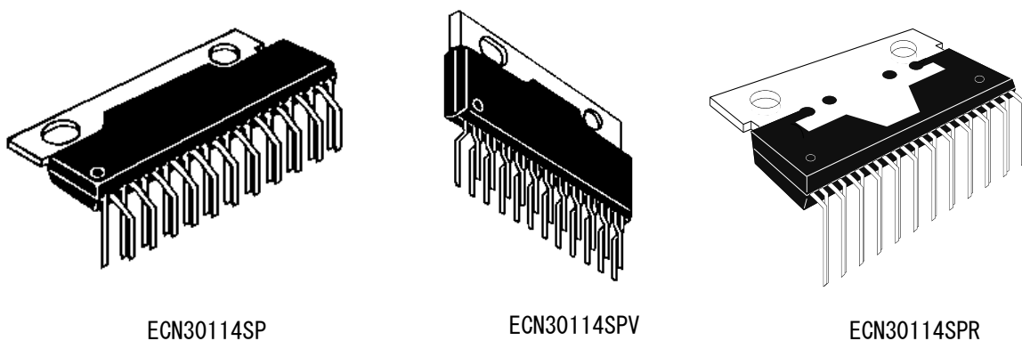
図1.4.1 EGN30114の外形
