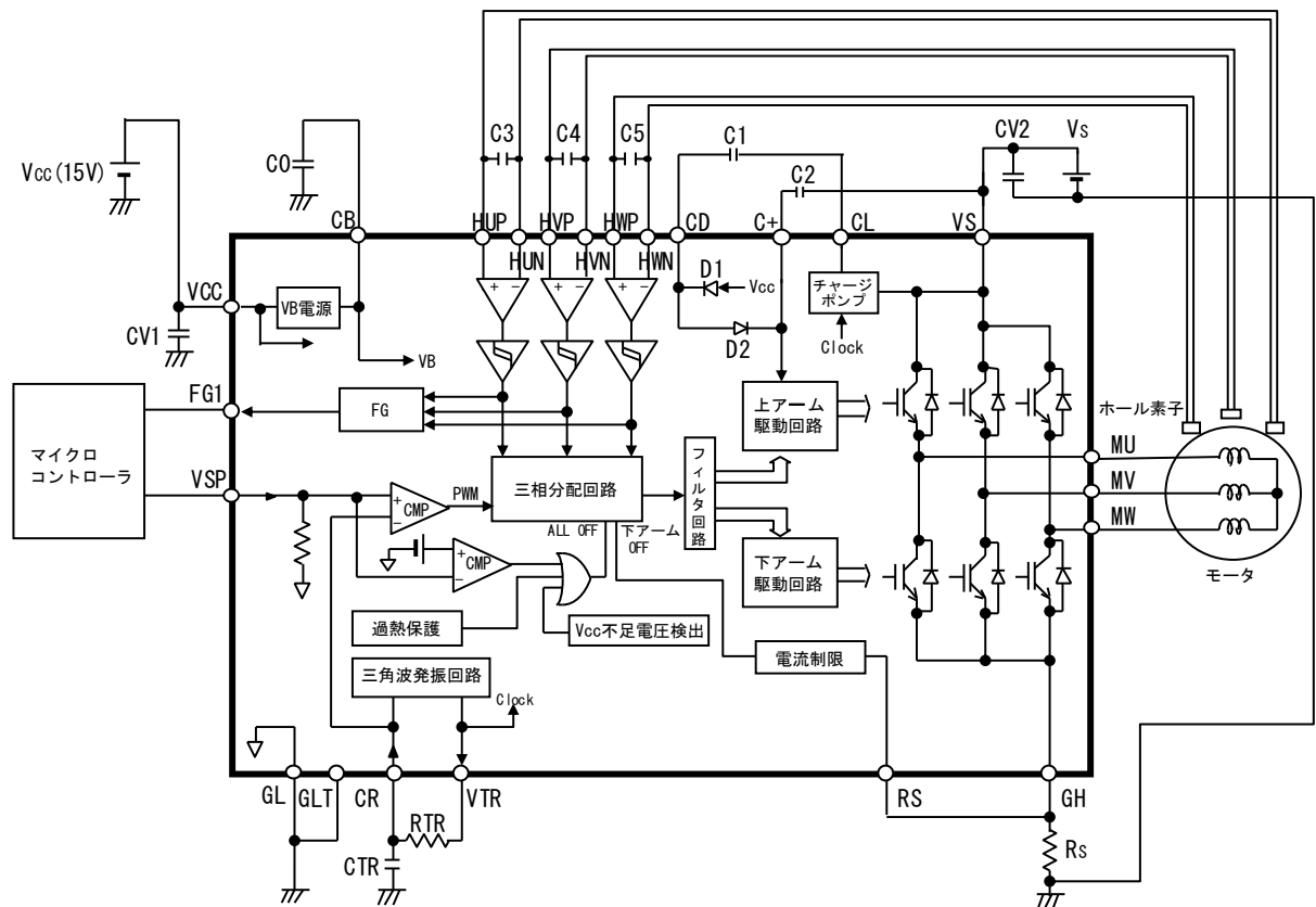
図 3.1.1 回路ブロック (太枠内 EGN30114)
