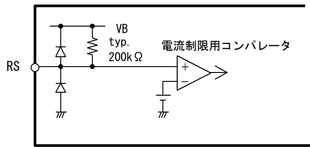
図 2. 2. 4 RS 端子の等価回路
