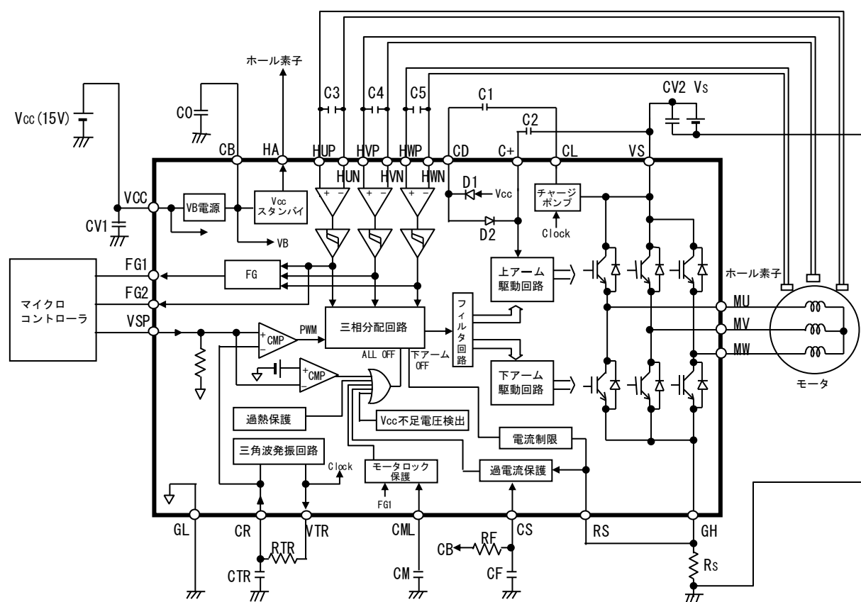
図 3.1.1 回路ブロック (太枠内 EGN30110)
