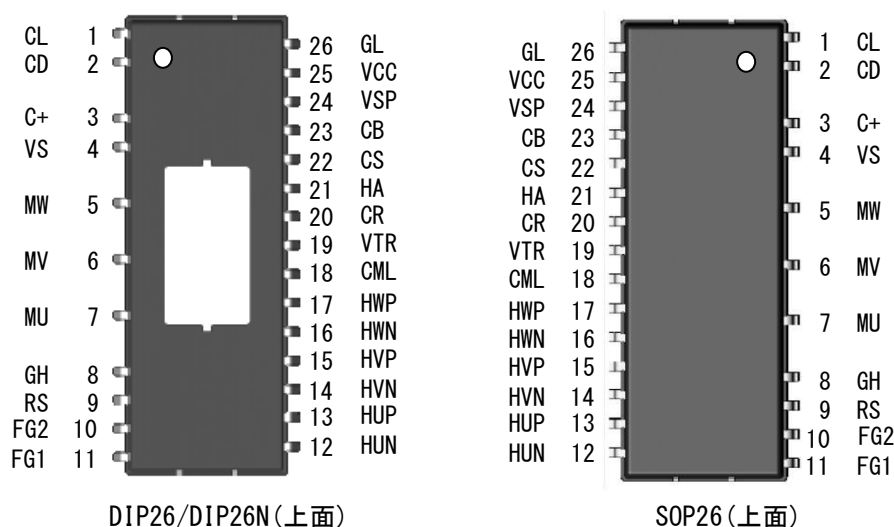
図5.1 端子配置
